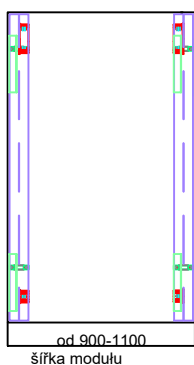
Vertikální řez
