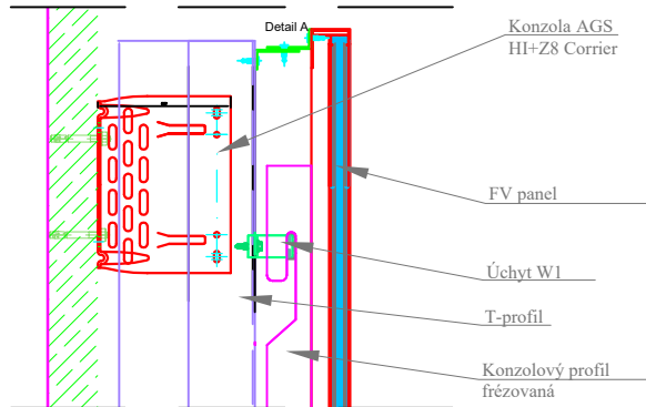
Vertikální řez
