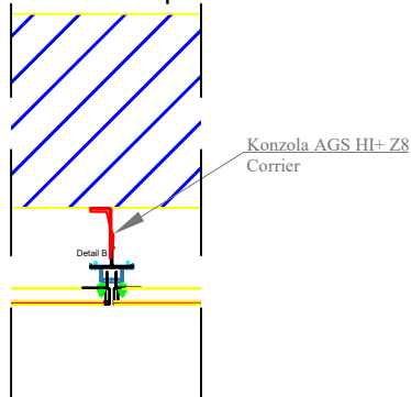
Horizontální průřez
